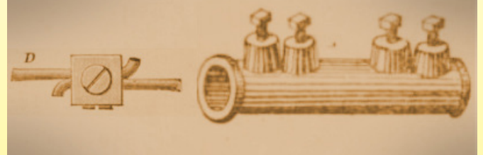
1892 Terminali a vite (Manuel pratique de l'installation de la lumière électrique. Impianti privati, di J.-P. Anney)
