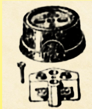
Presi di corrente con base in porcellana e coperchio in bachelite (Maure Catalog 1932, Ultimheat Museum)
