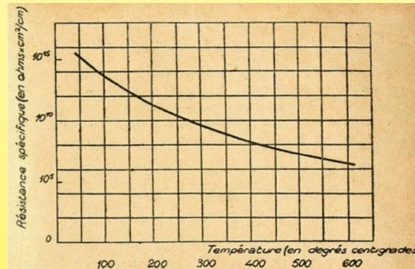
Variazione della resistenza specifica in ohm.cm/cm 2 della porcellana in funzione della temperatura (curva logaritmica). Tra 20°C e 300°C la sua resistenza è divisa per 10,000 (1945 Matériaux électrotechniques modernes, Ultimheat Museum).
